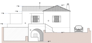
ΣΧΗΜΑΤΙΚΕΣ ΟΡΕΣ
