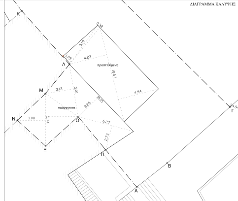
ΔΙΑΓΡΑΜΜΑ ΚΑΛΥΨΗΣ
